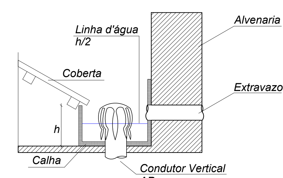
DETALHE DO EXTRAVAZOR ESCALA _____ 10
